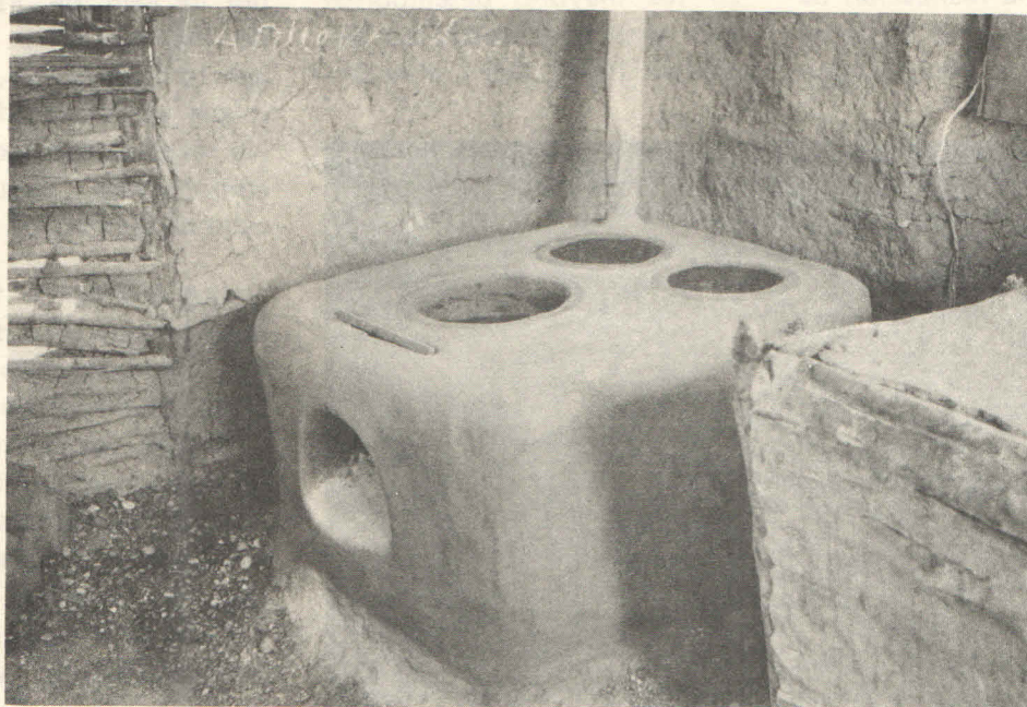
Un modelo de las estufas lorenas que MUDE ayuda a construir en comunidades de Azua, al Sur del país.
